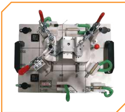
Đồ gá kiểm tra (sheet metal checking fixture)
