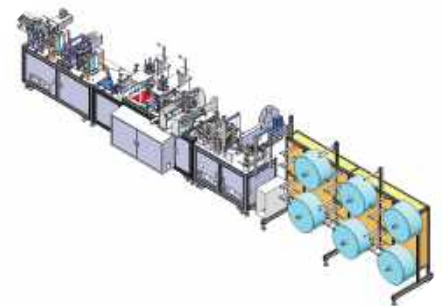
Máy khâu trang (Mask Making Machine)
