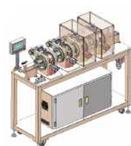
Máy uốn linh kiện ( Auto terminal bending Machine)
