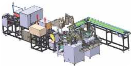
Dây chuyền kiểm tra (Auto Inspection Line)
