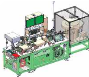
Dây chuyền lắp ráp - kiểm tra linh kiện (Auto Assem-Inspection Line)
