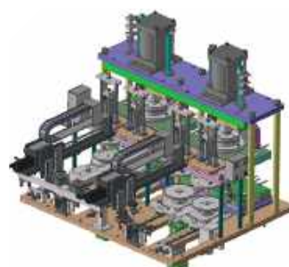
Máy ép nhiệt bôi keo (Glue-Thermal press Machine)
